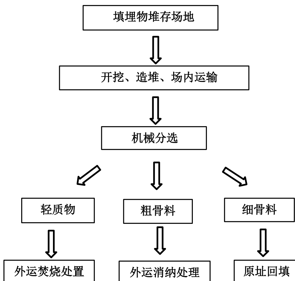
处理方案总工艺流程图
